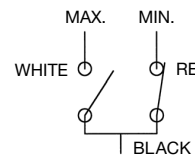
LEM5MA MIN. - MAX. CONTACTS
