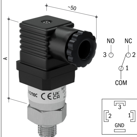
Conector DIN 43650 PG09 DIN 43650 PG09 connector
