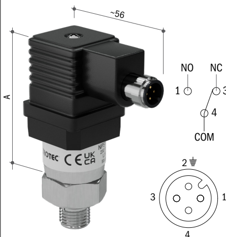
Adaptador DIN 43650 A a M12 DIN 43650 A to M12 adaptor
